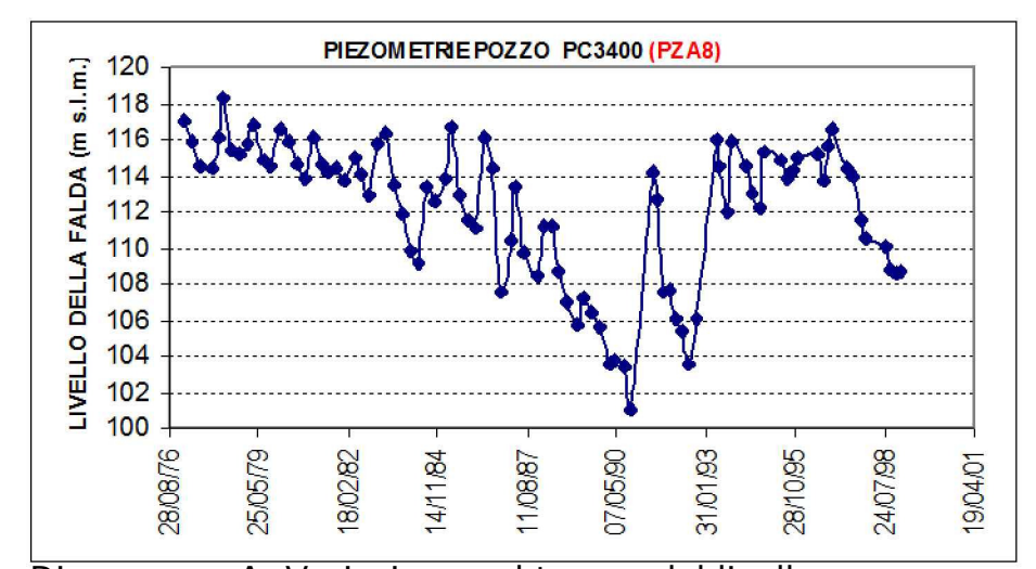
Diagramma A. Variazione nel tempo del livello piezometrico (Gruppi acquiferi A1-C1). Località Lusurasco; profondità pozzo 101.0 m
