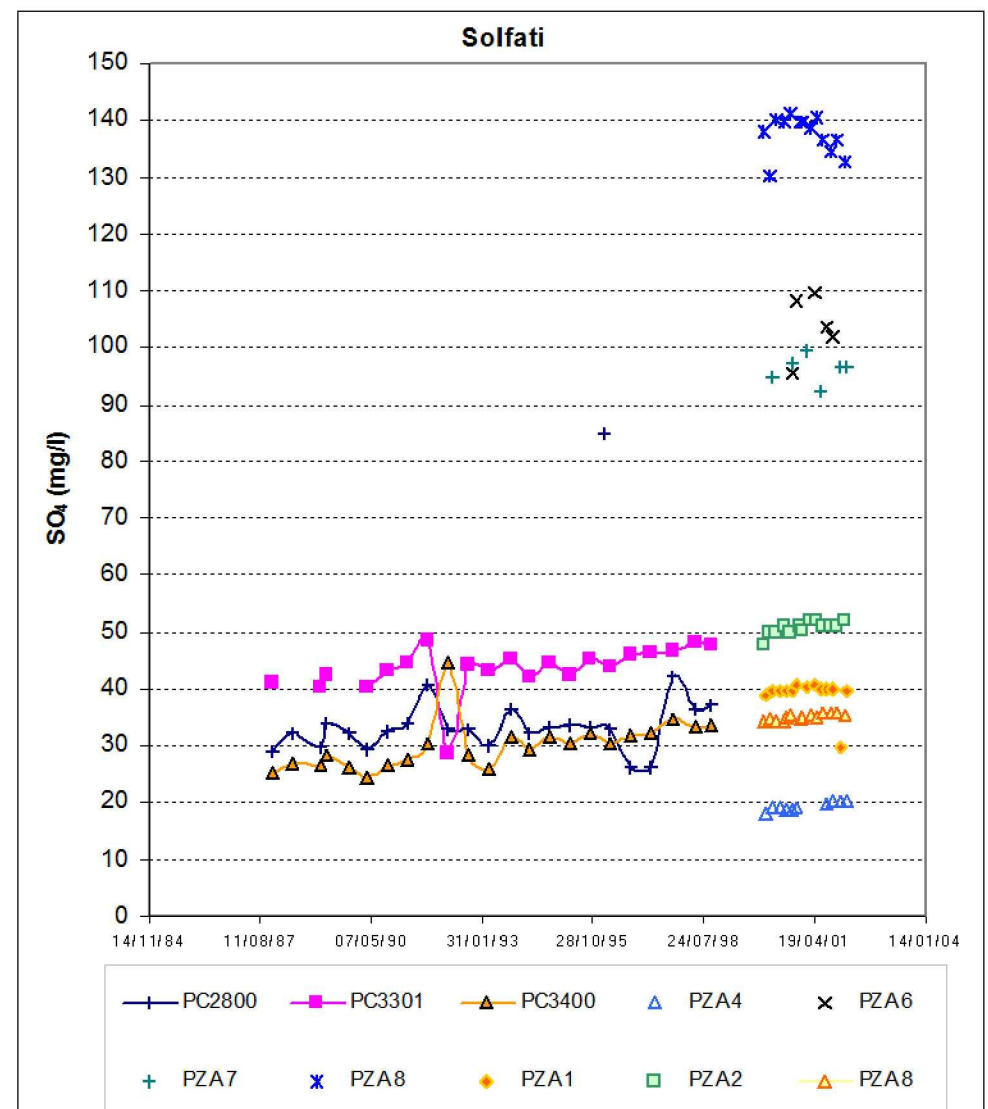
Diagramma C. Concentrazione dei solfati nei pozzi monitorati
