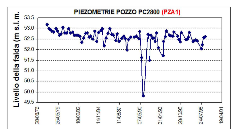
Diagramma B. Variazione nel tempo del livello piezometrico (Gruppi Acquiferi A1 e A2). Località Chiaravalle della Colomba; profondità pozzo 60.0 m.
