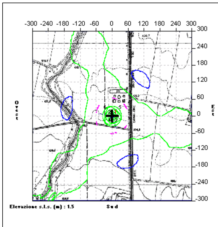
FIGURA 2: sezione orizzontale del campo elettrico a 1.5 m dal suolo
