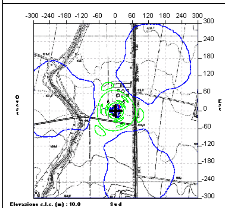
FIGURA 3: sezione orizzontale del campo elettrico a 10 m dal suolo
